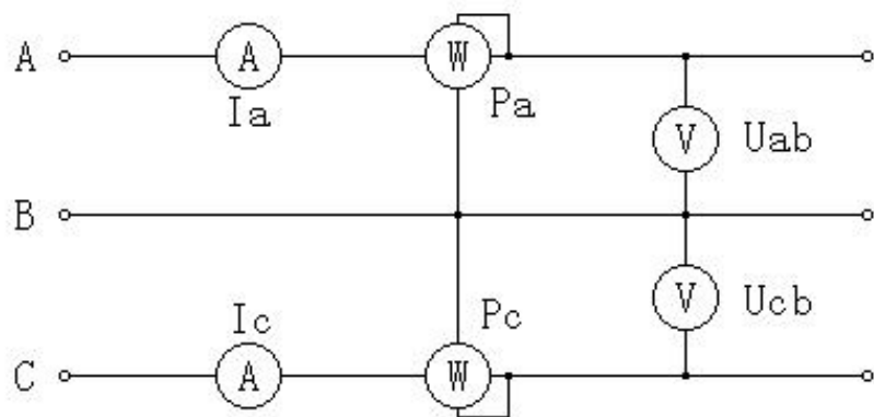
图十七、三相三线计量原理图
