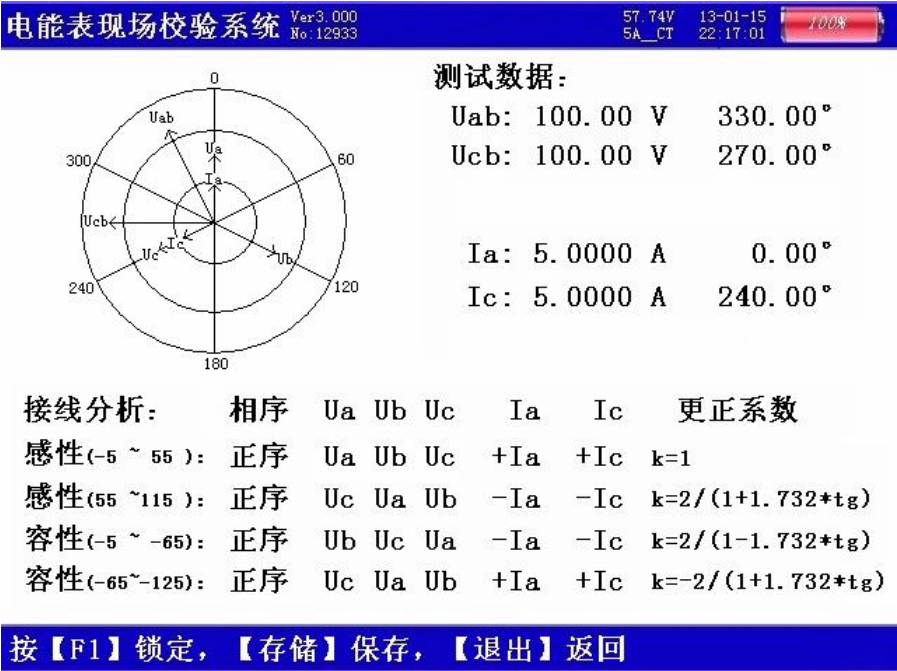
图十、矢量分析屏一三相三线
