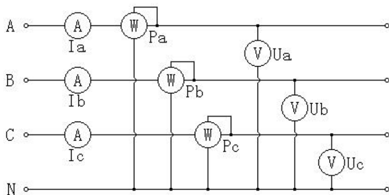
图十八、三相四线计量原理图
